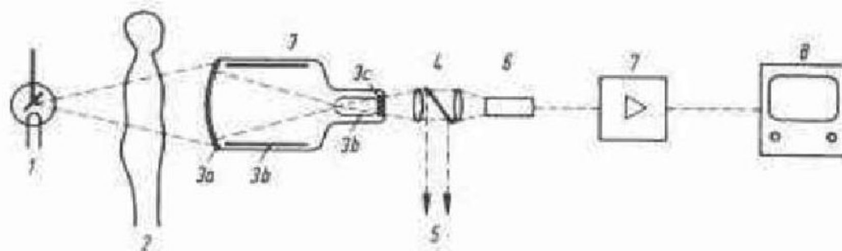
图8 影像增强屏系统
