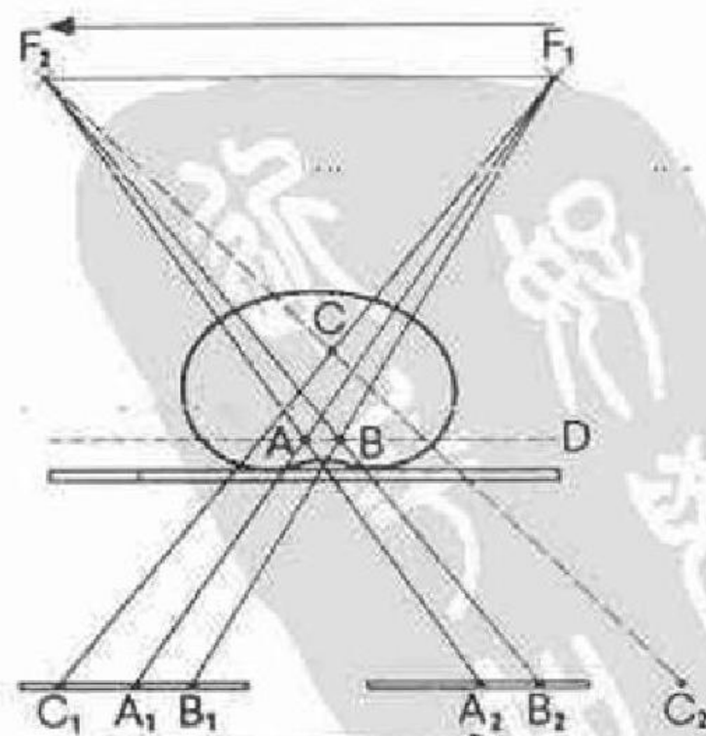
图6 断层成像示意图
