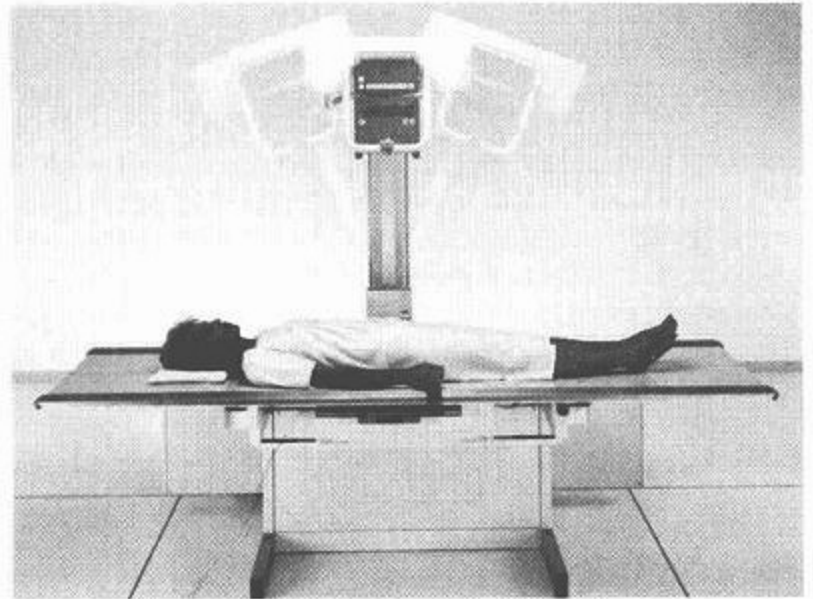
图5 带有可平移式检查床的断层扫描仪
