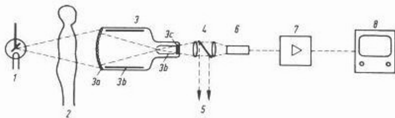
图8 影像增强屏系统
